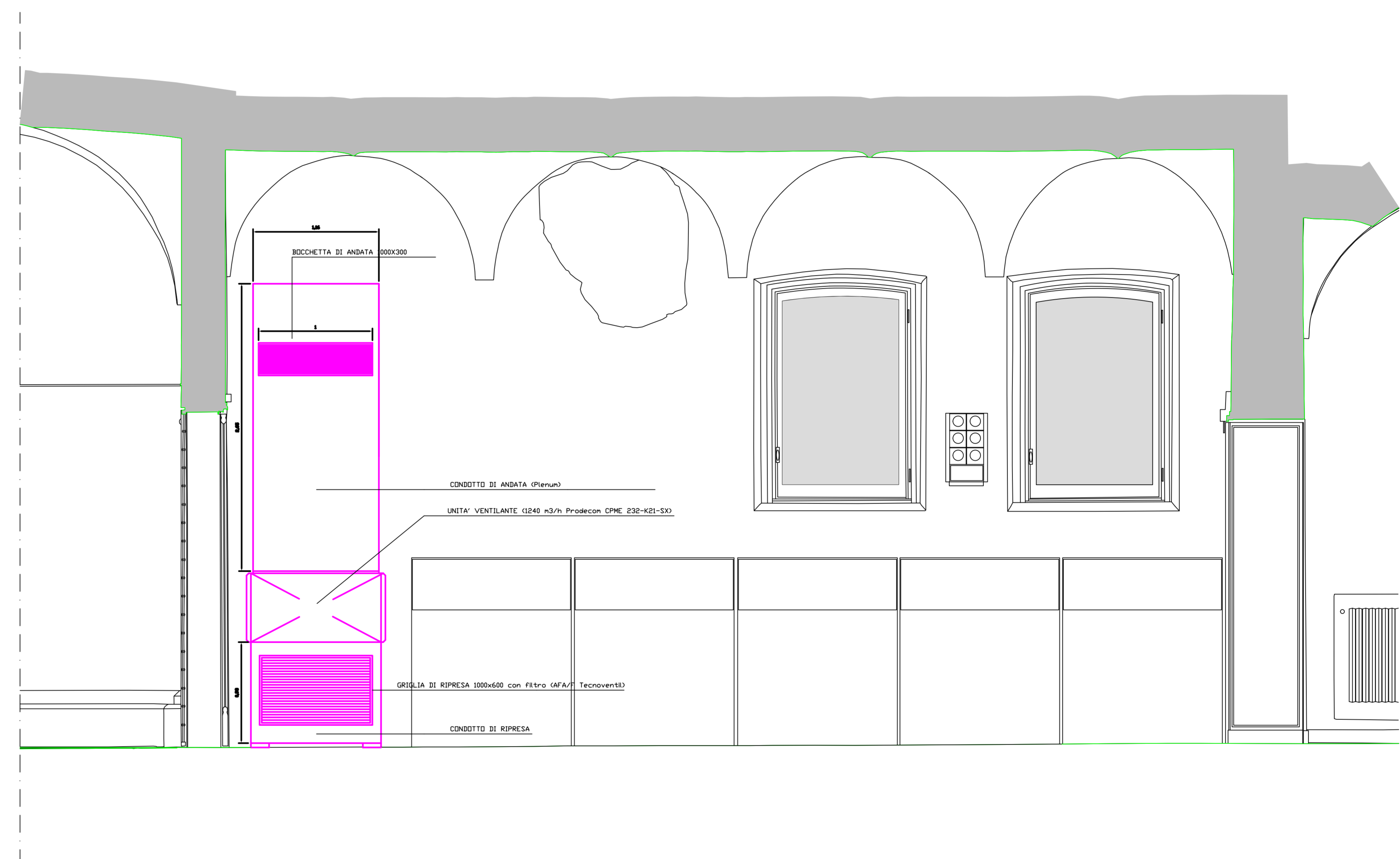
SEZIONE I-I
